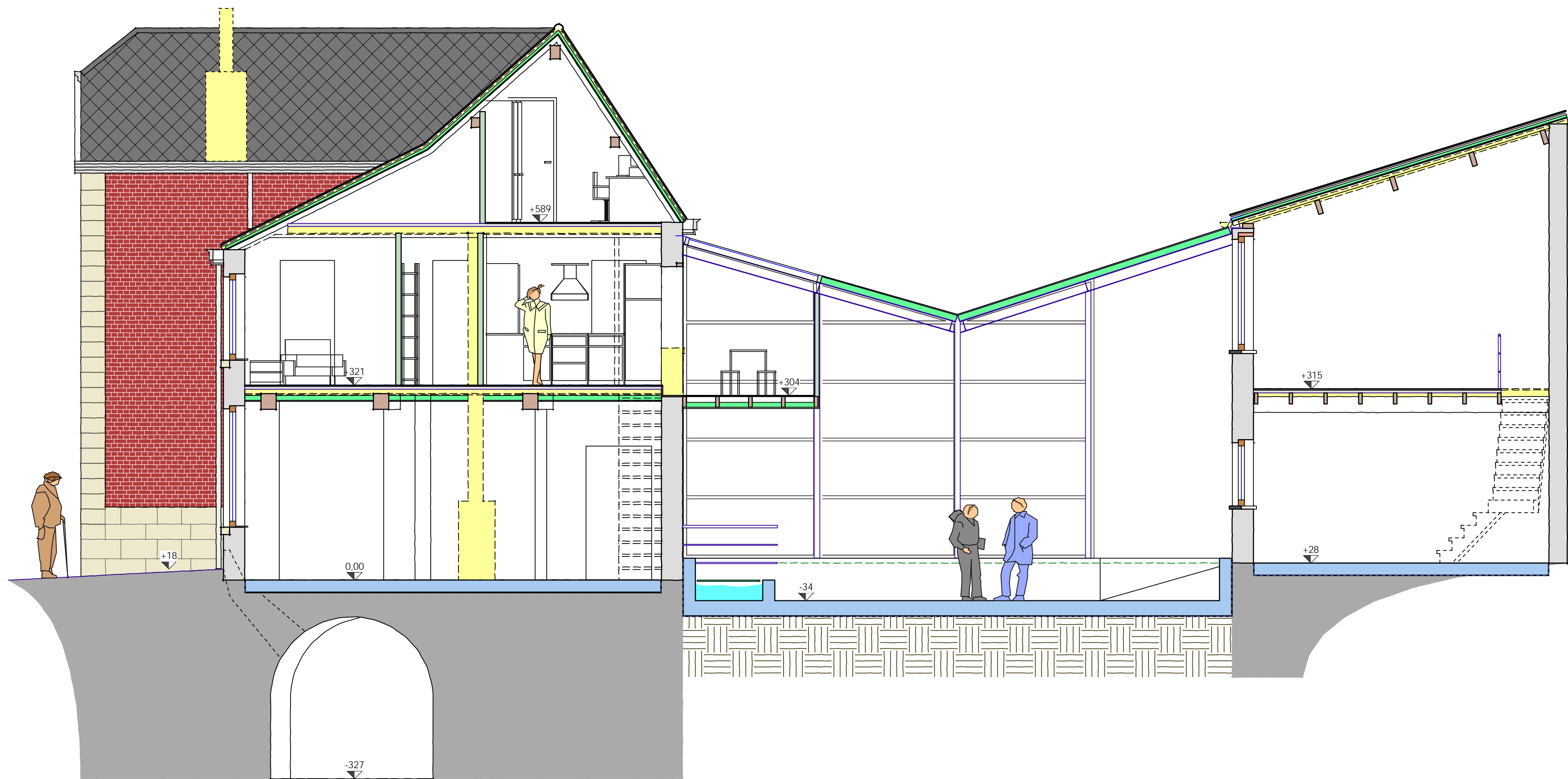
Doorsnede C
